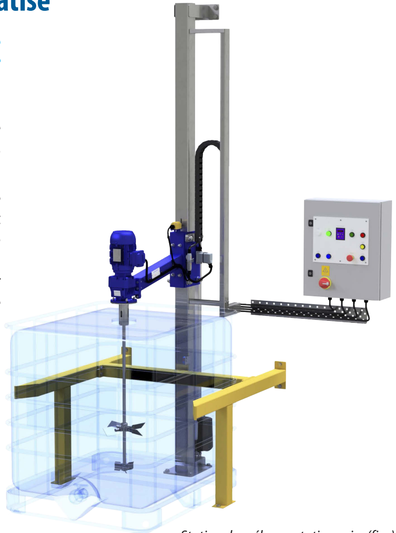
Station de mélange stationnaire (fixe)
